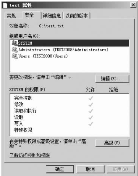
图 3-1 查看 NTFS 权限
