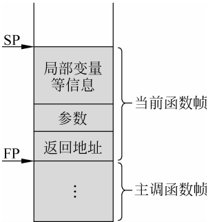
图 3-24 栈帧结构
