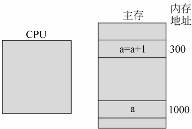
图 3-1 计算机执行 a=a+1 语句
