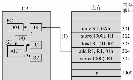
图 3-7 执行 add 指令
