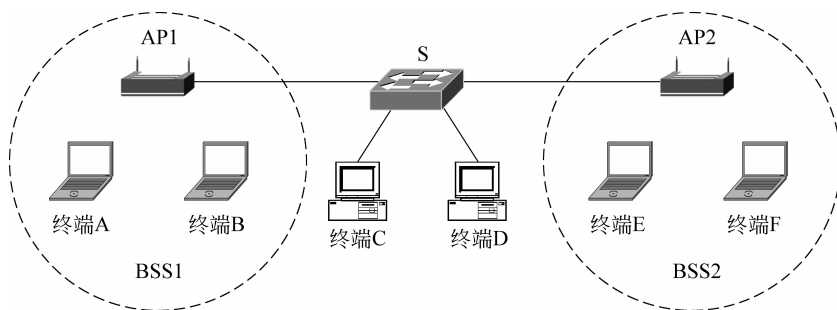
图 5.1 无线局域网结构
