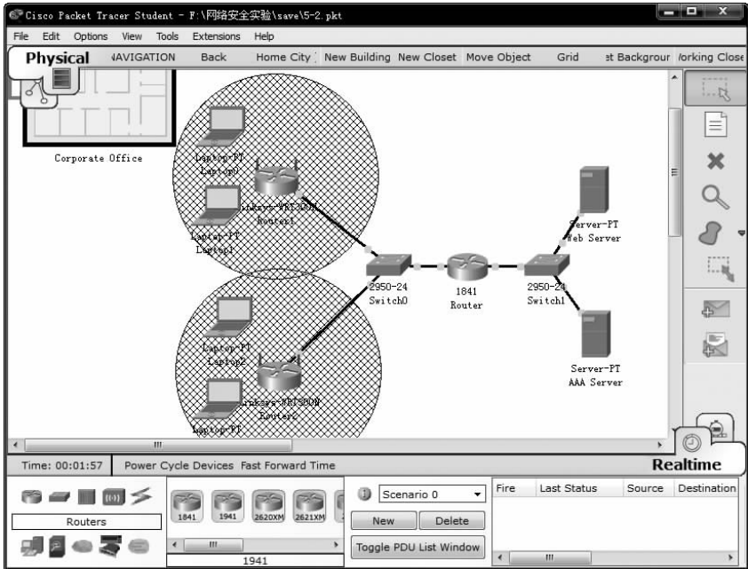
图 5.12 完成设备放置和连接后的物理工作区界面
