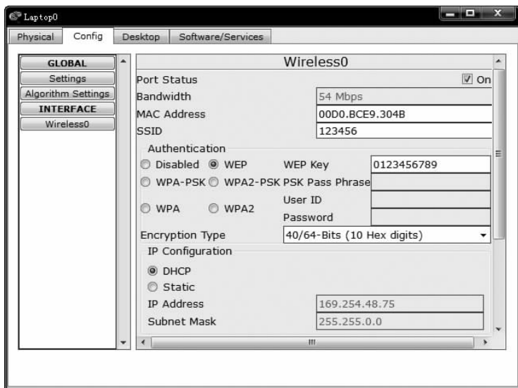
图 5.5 Laptop0 与实现 WEP 安全机制相关参数的配置过程
