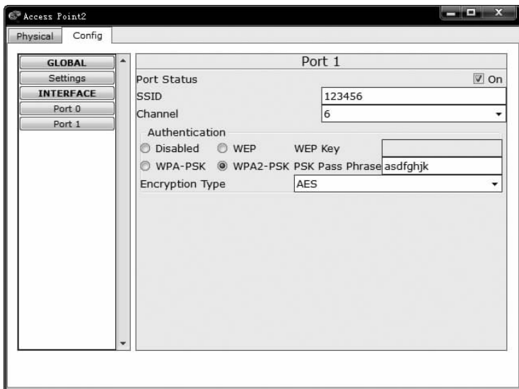
图 5.6 AP 与实现 WPA2-PSK 安全机制相关参数的配置过程
