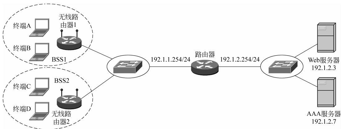
图 5.10 无线局域网结构
