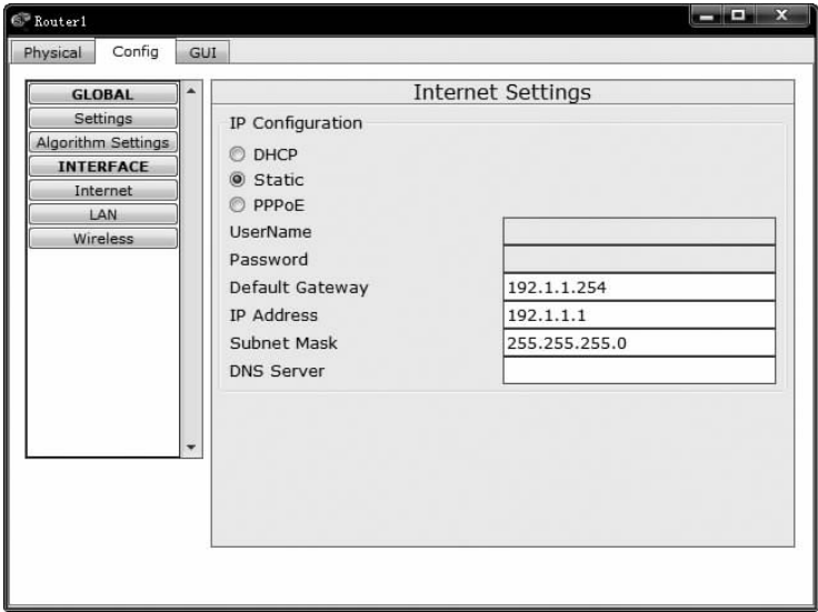
图 5.15 无线路由器 Router1 Internet 接口配置界面
