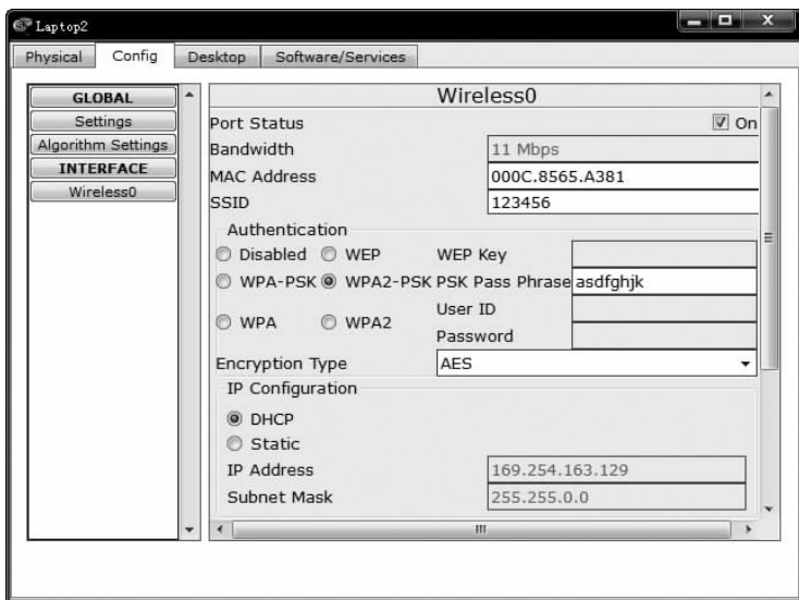
图 5.7 Laptop2 与实现 WPA2-PSK 安全机制相关参数的配置过程
