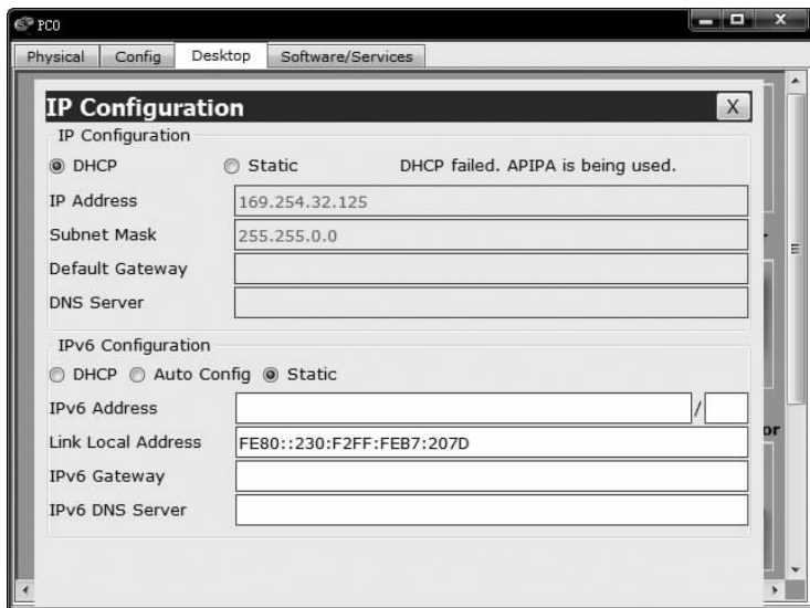
图 5.9 PC0 自动获取网络信息过程
