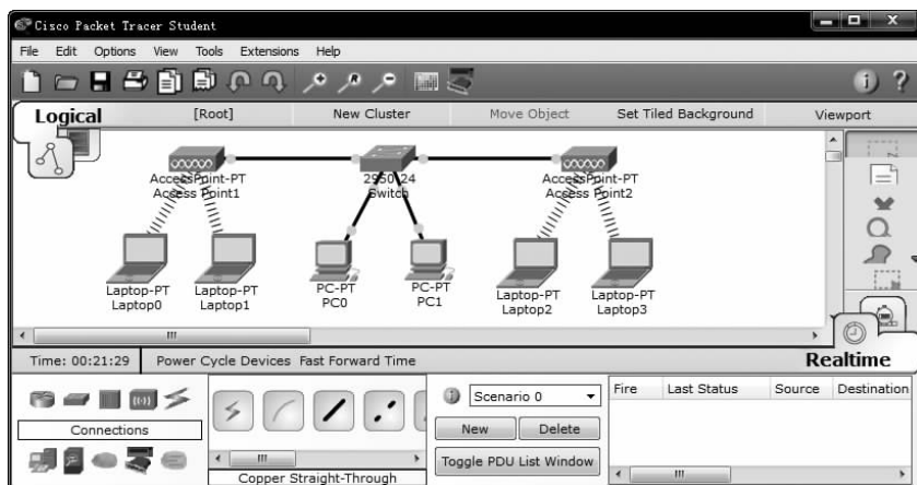
图 5.8 笔记本电脑与 AP 之间成功建立关联后的逻辑工作区界面
