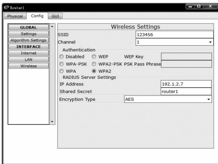
图 5.14 无线路由器无线接口配置界面
