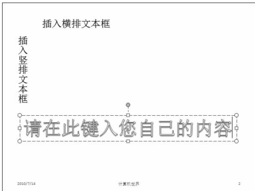
图 5-20 插入艺术字
