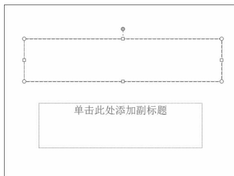
图 5-12 选定标题框
