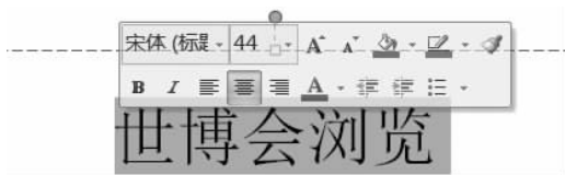
图 5-2 浮动工具栏
