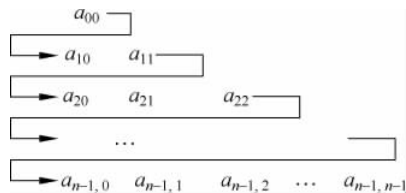
图 5.3 对称矩阵的行优先存放
