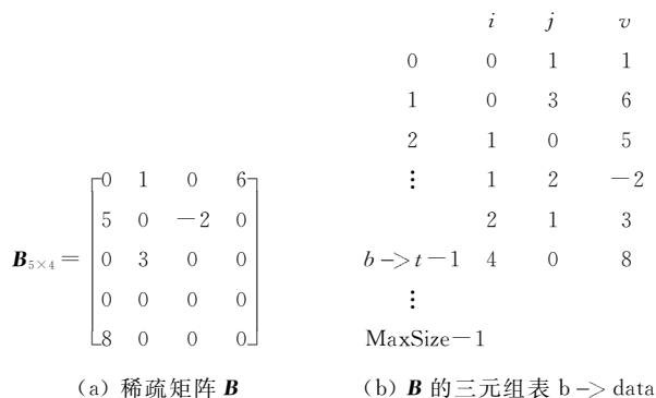
图 5.7 稀疏矩阵 \mathbf{B} 和它的三元组表 *b
