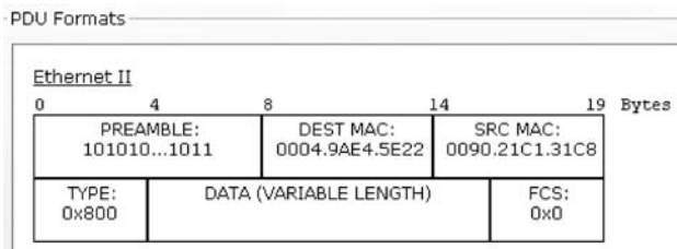
图 3-9 Packet Tracer 中查看以太网帧结构示例
