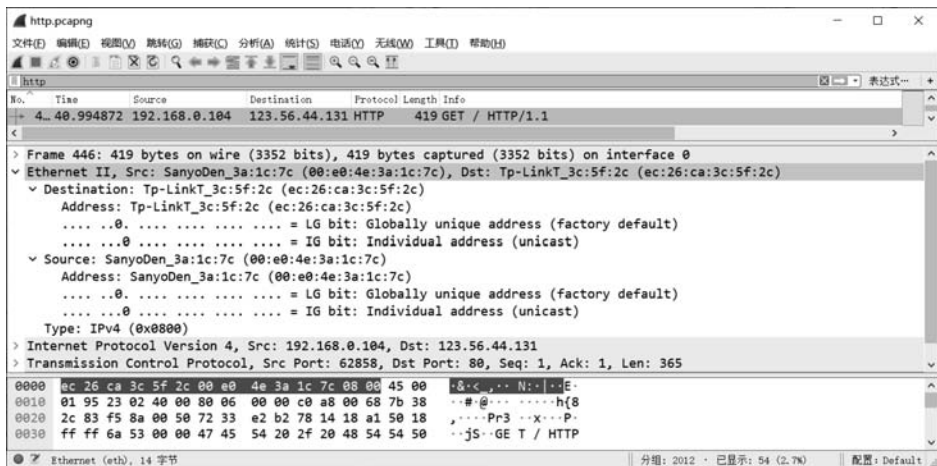
图 3-6 以太网帧结构分析示例
