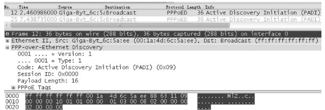
图 3-14 拨号上网的 PPPoE 帧结构示例
