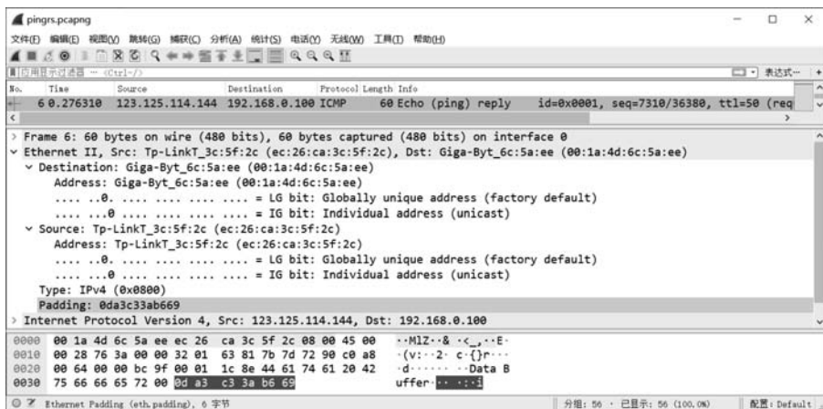
图 3-7 包含 Padding 字段的以太网帧示例
