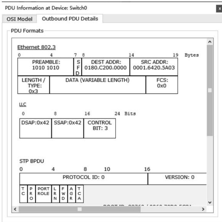
图 3-10 IEEE 802 帧结构示例
