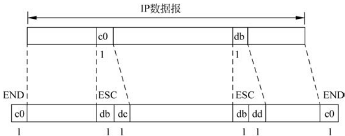
图 3-3 SLIP 报文的封装结构
