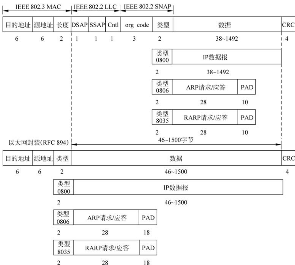
图 3-2 IEEE 802.2/IEEE 802.3(RFC1042)和以太网(RFC 894)的封装格式
