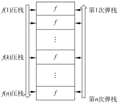
图 3.4 递归过程中最长栈的长度是 n
