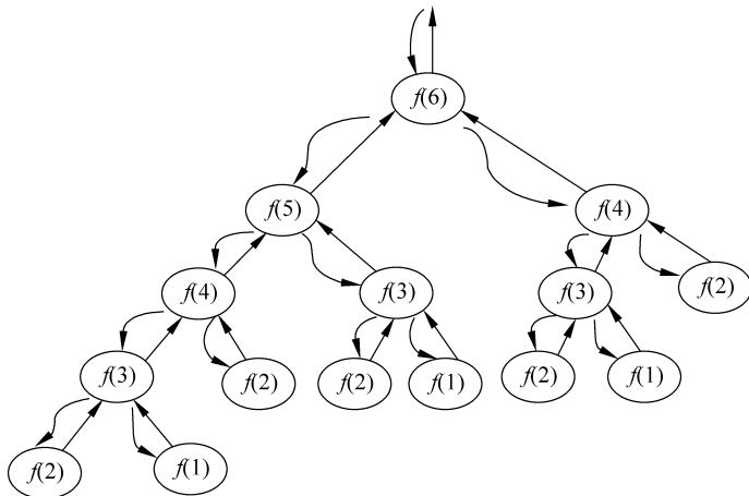
图 3.6 递归过程的二叉树示意图
