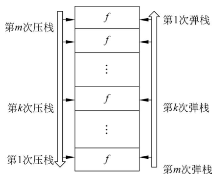
图 3.2 递归过程中的压栈、弹栈
