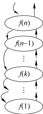
图 3.3 递归过程中函数的调用和结束
