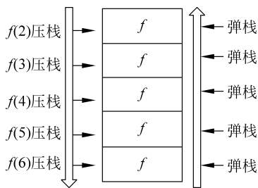
图 3.7 递归过程中的最长栈
