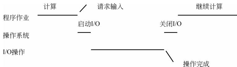
图 3.4 单道程序工作示例
