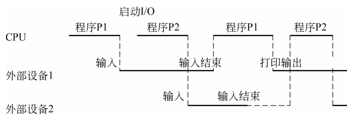
图 3.5 多道程序工作示例
