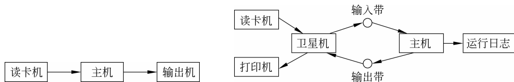
图 3.2 脱机处理系统
