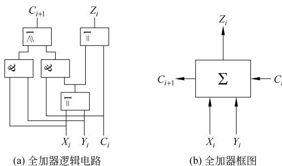
图 3.1 一位全加器逻辑及其框图
