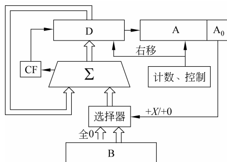
图 3.6 原码一位乘法器框图
