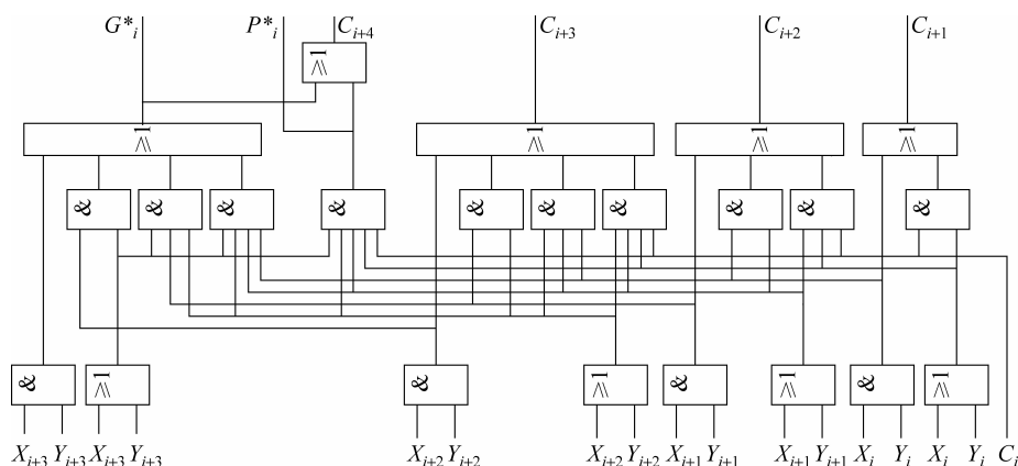
图 3.3 四位先行进位链电路
