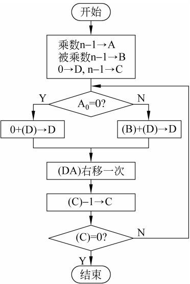
图 3.4 绝对值乘法思路框图
