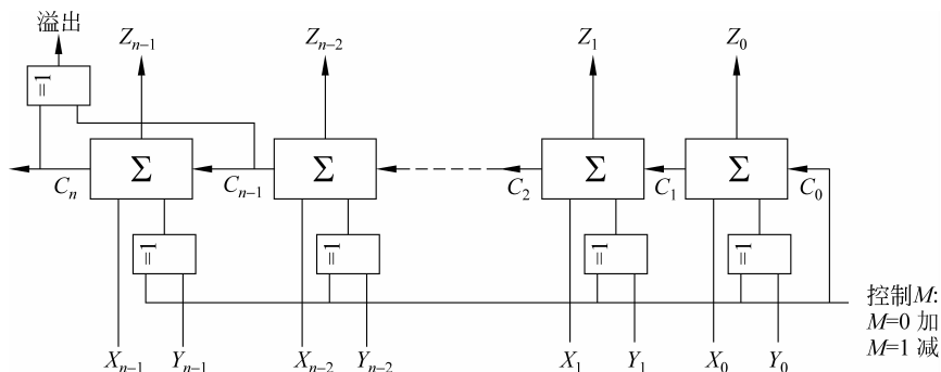
图 3.2 行波进位的 n 位加法/减法器
