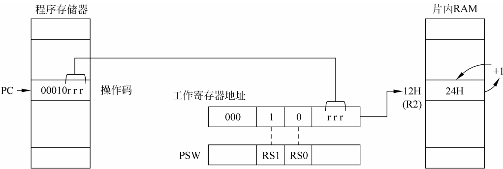
图 3-1 寄存器寻址方式
