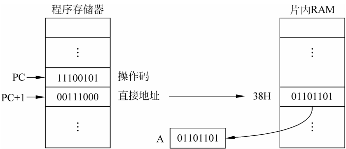
图 3-2 直接寻址方式
