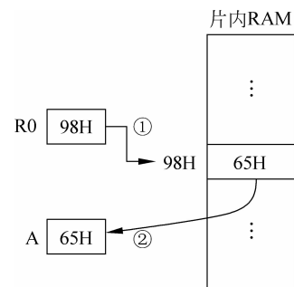
P2 中的值作为高 8 位地址,Ri 中的值作为低 8 位地址。图 3-3 间接寻址(MOV A, @R0)示意图 P2 为 0 时,访问的区域为 pdata。
