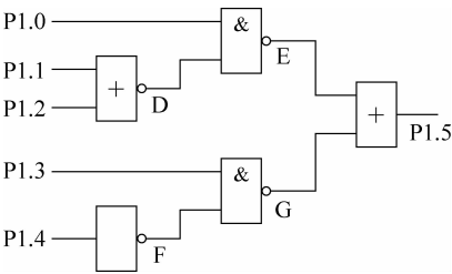
图 3-5 硬件逻辑电路
