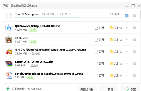
图 1.12 下载软件
