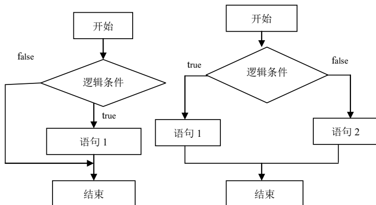
图 5-2 单向选择和双向选择结构
