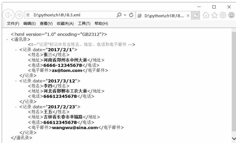
图 18-5 元素包含数据
