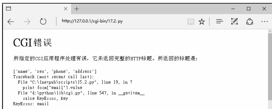
图 17-3 程序运行结果
