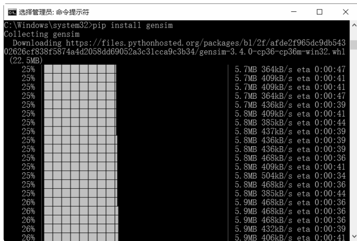
图 22-3 安装 gensim 库
