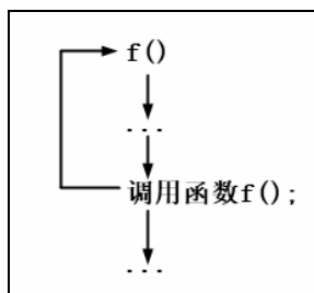
图 6-39 递归过程
