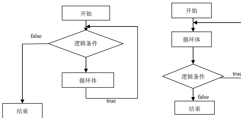
图 5-3 循环结构
