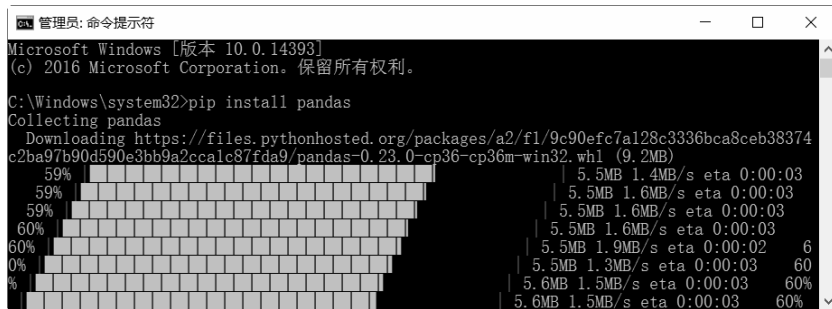
图 21-2 安装 pandas 库
