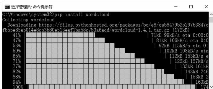
图 22-4 安装 wordcloud 库
