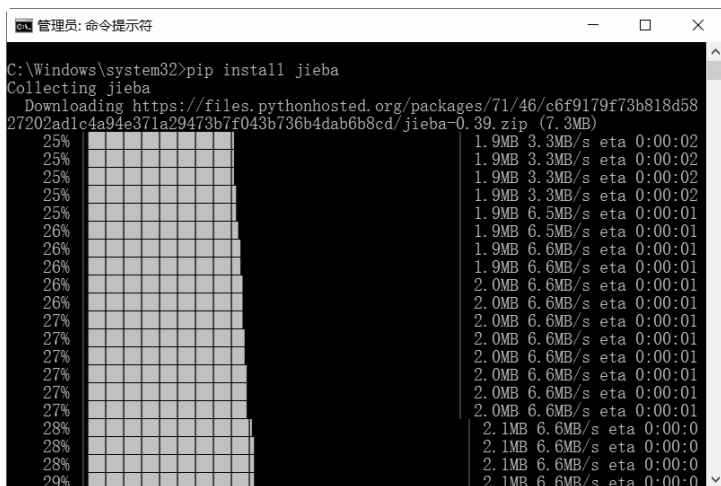
图 22-2 安装 jieba 库
