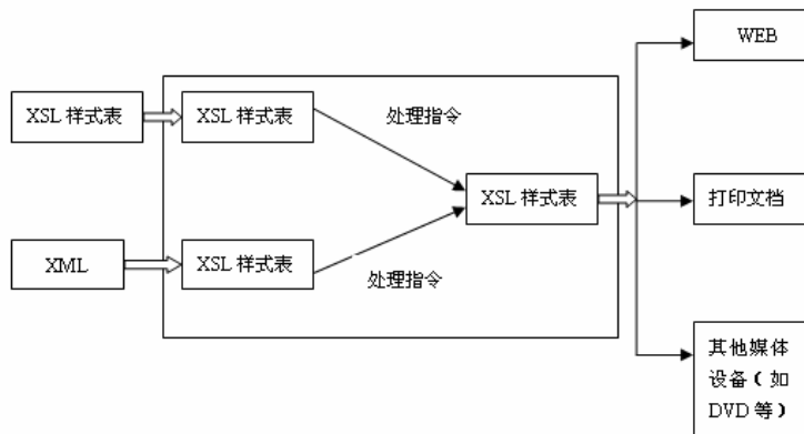
图 18-1 XSLT 转换过程
