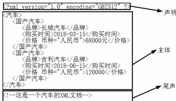
图 18-3 XML 文档组成
