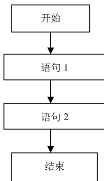
图 5-1 顺序结构
