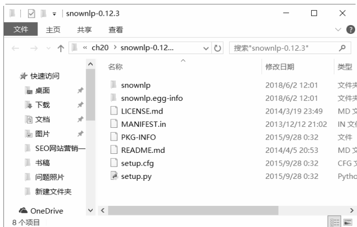
图 20-3 解压文件
