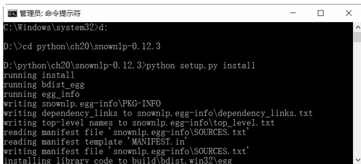
图 20-4 安装 snownlp 库
