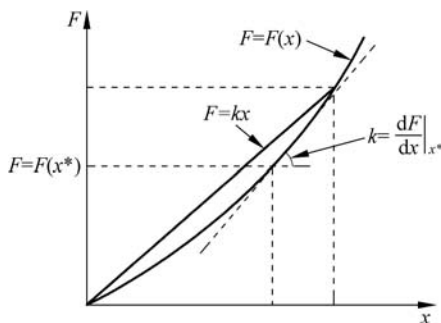
图 1-10 弹簧力与变形的关系
