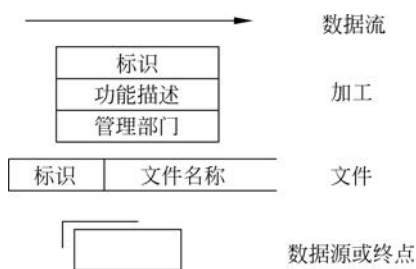
图 3.14 数据流图的基本符号
