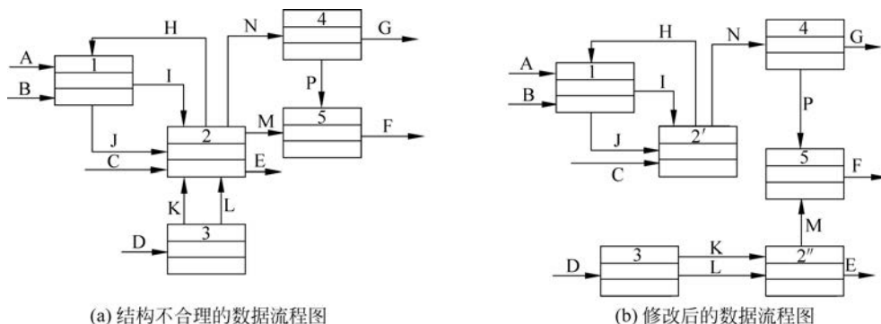
图 3.22 结构不合理的数据流程图及其修改
