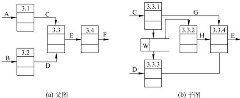
图 3.20 数据流图中的局部文件
