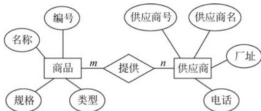
图 3.10 实体、实体属性及实体联系模型图
