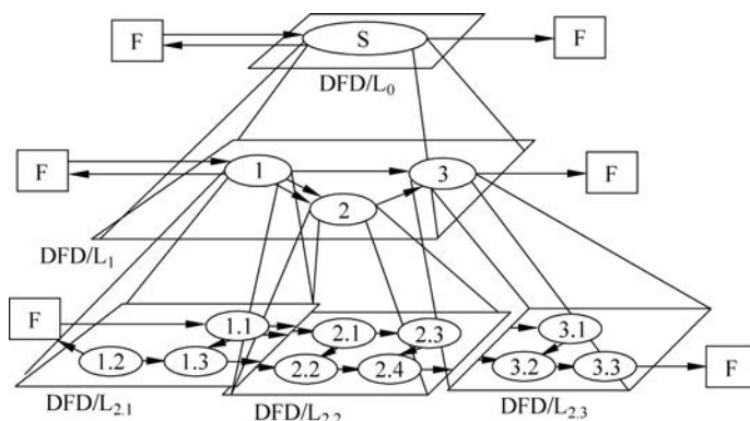
图 3.13 分层数据流图
