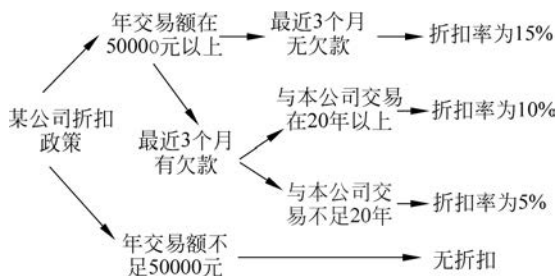
图 3.28 判定树描述的折扣政策
