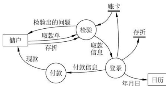
图 3.11 办理取款手续的数据流程图
