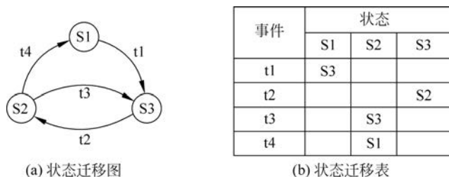
图 3.23 状态迁移图及与其等价的状态迁移表
