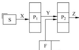
图 3.15 数据流图举例
