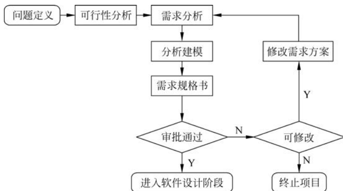
图 3.1 系统分析过程流程图
