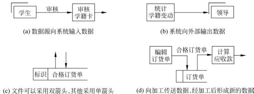
图 3.16 常见的几种可能的数据流
