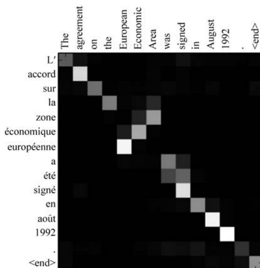
图 5-5 Attention 结果可视化
