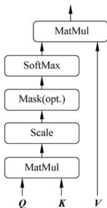
图 5-6 Self-Attention 的计算过程
