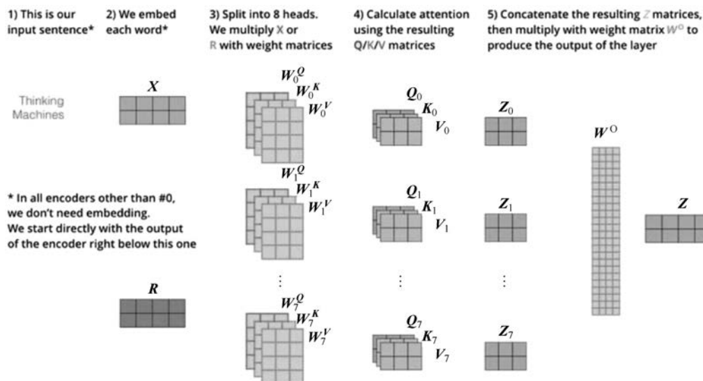
图 5-11 Multi-Head Attention 计算
