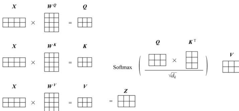
图 5-9 矩阵形式
