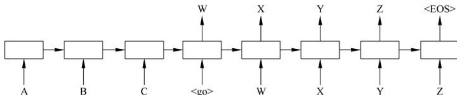
图 5-1 Encoder-Decoder
