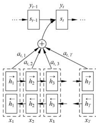
图 5-4 Attention 机制
