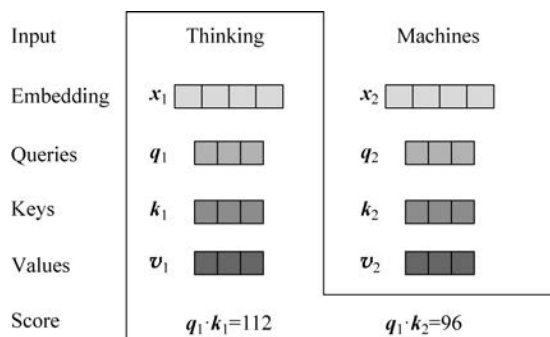
图 5-7 Attention 计算(1)
