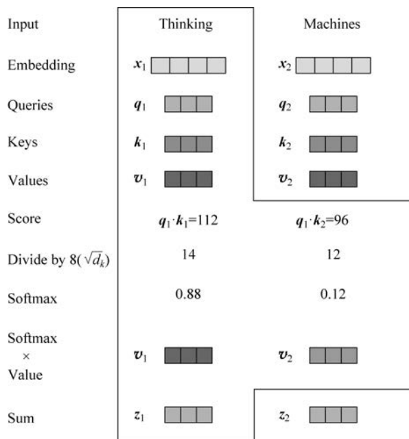
图 5-8 Attention 计算(2)
