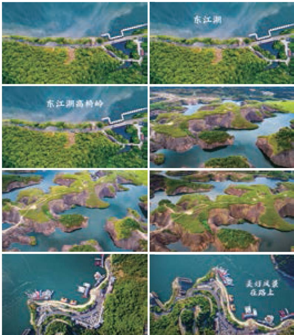
图1-1 画面效果
