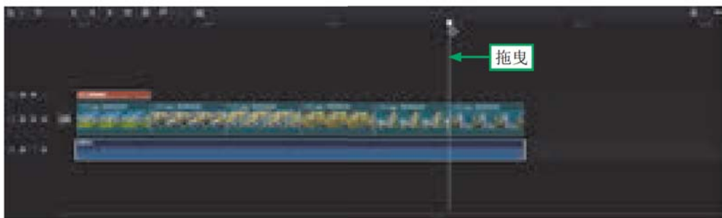
图1-19 拖曳时间轴
