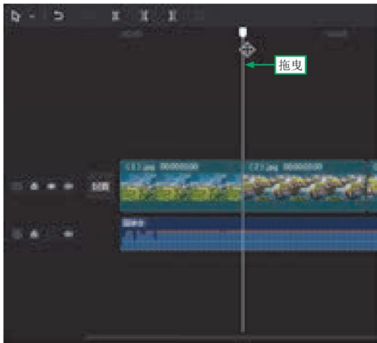
图1-11 拖曳时间轴
