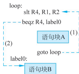
图 3-14 用汇编指令表述 while 循环语句的执行
