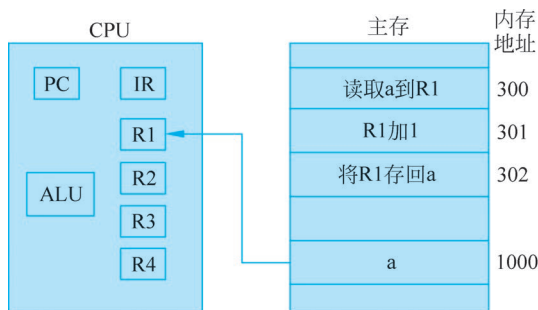
图 3-4 load 指令
