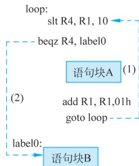
图 3-16 汇编指令表述 for 循环的执行
