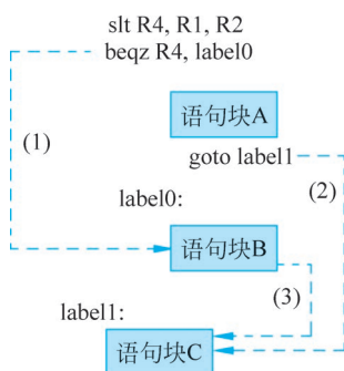
图 3-9 用汇编指令表述 if-else 的执行
