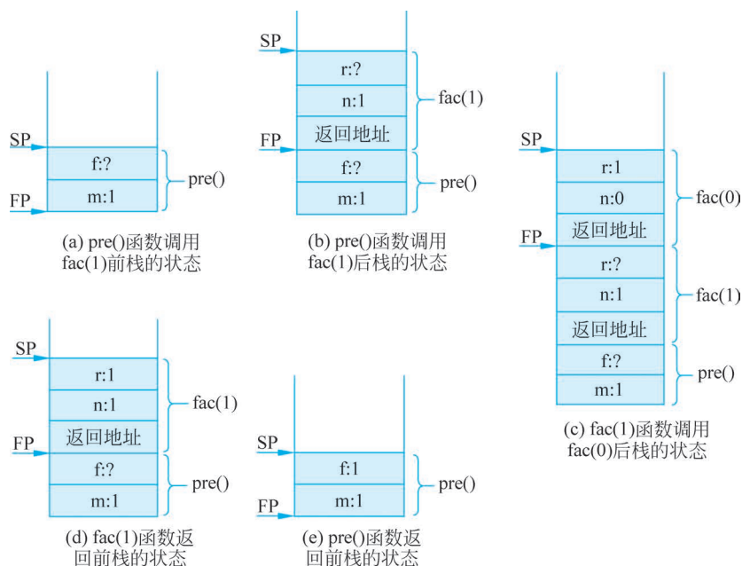
图 3-26 递归函数调用过程中的栈示意图
