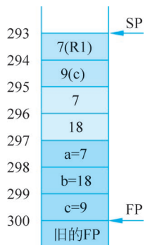
图 3-35 第二次函数调用传参后栈的状态
