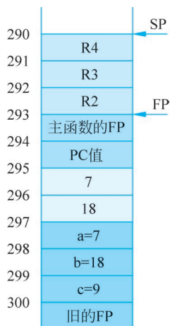
图 3-33 push 需要保护的寄存器的值
