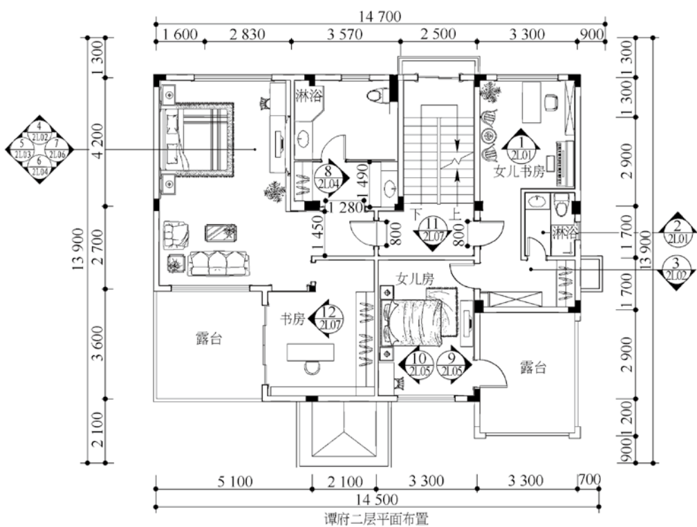
图 1-7 别墅设计平面图 (文健、石树勇 设计)
