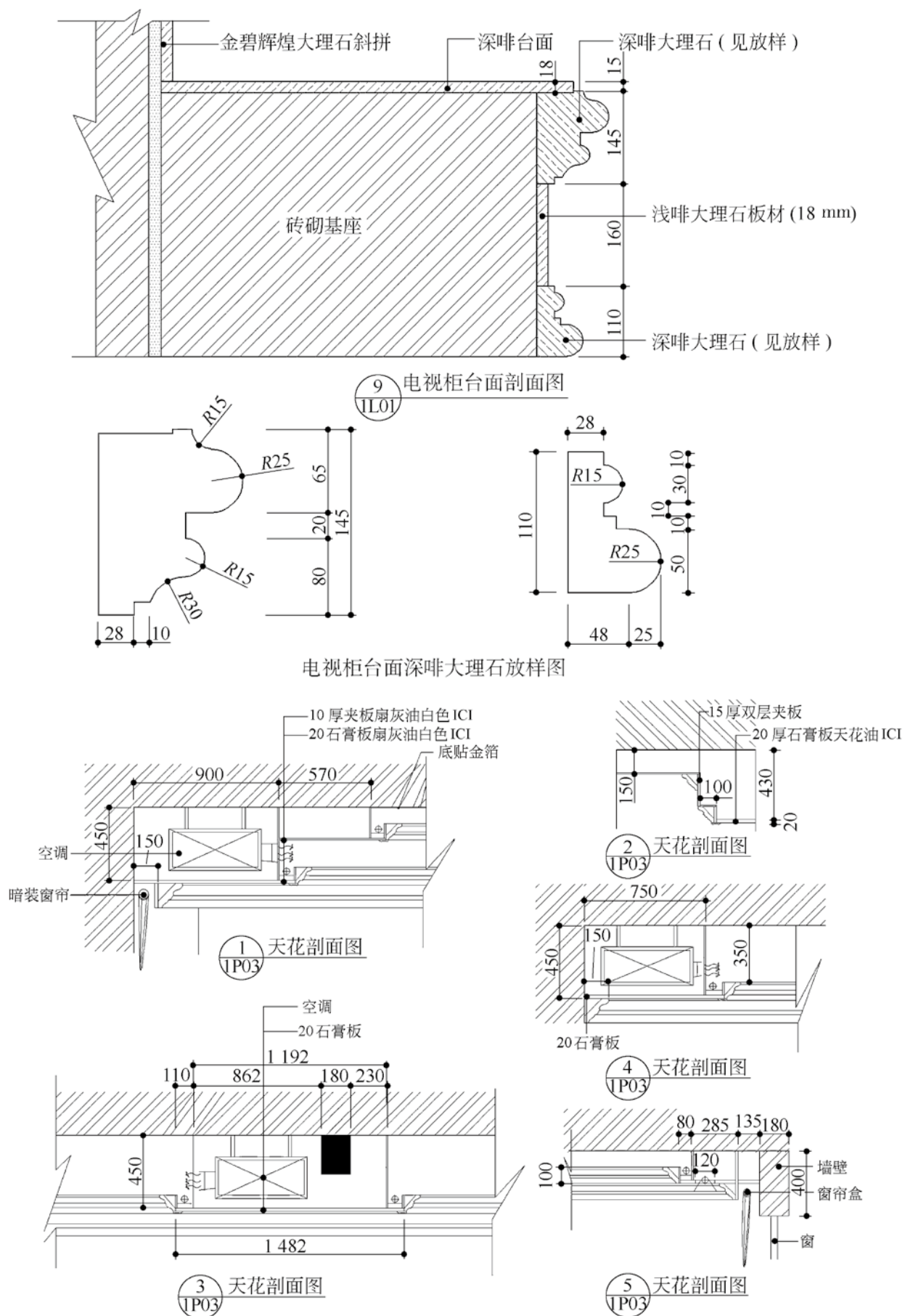
图 1-15 别墅设计剖面图 (2) (文健、石树勇 设计)
