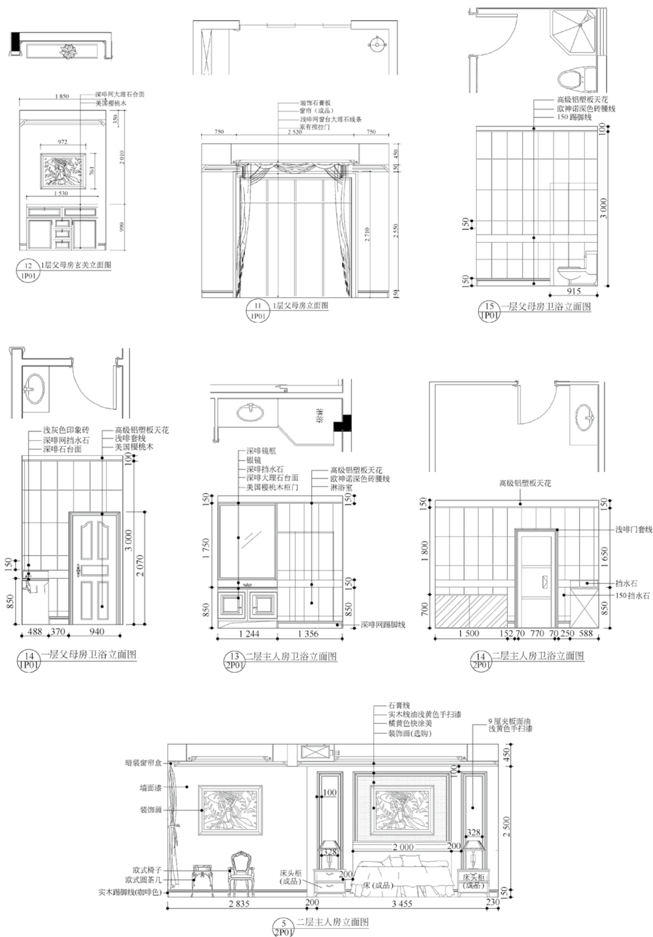
图 1-13 别墅设计立面图(3)(文健、石树勇 设计)
