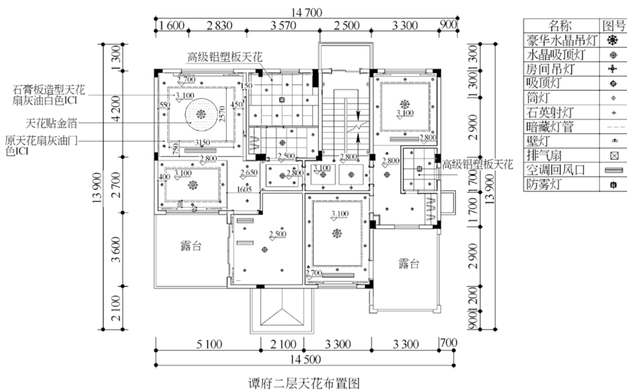
图 1-9 别墅设计天花图 (1) (文健、石树勇 设计)
