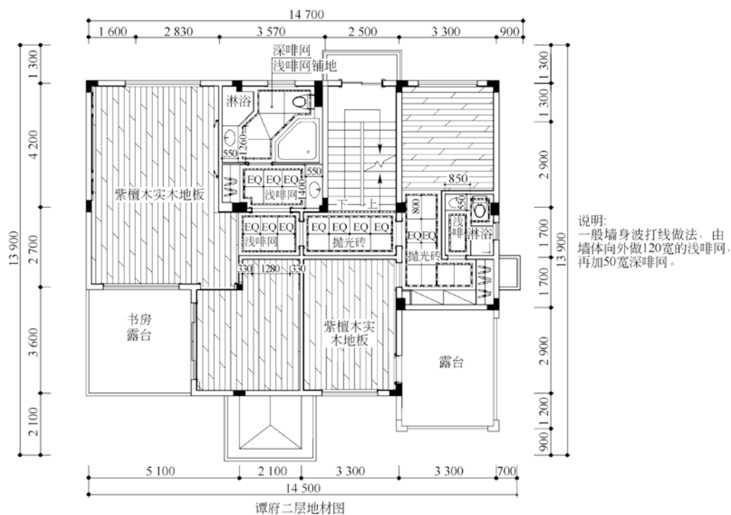
图 1-8 别墅设计地材图 (文健、石树勇 设计)
