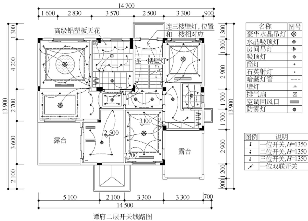
图 1-10 别墅设计天花图 (2) (文健、石树勇 设计)
