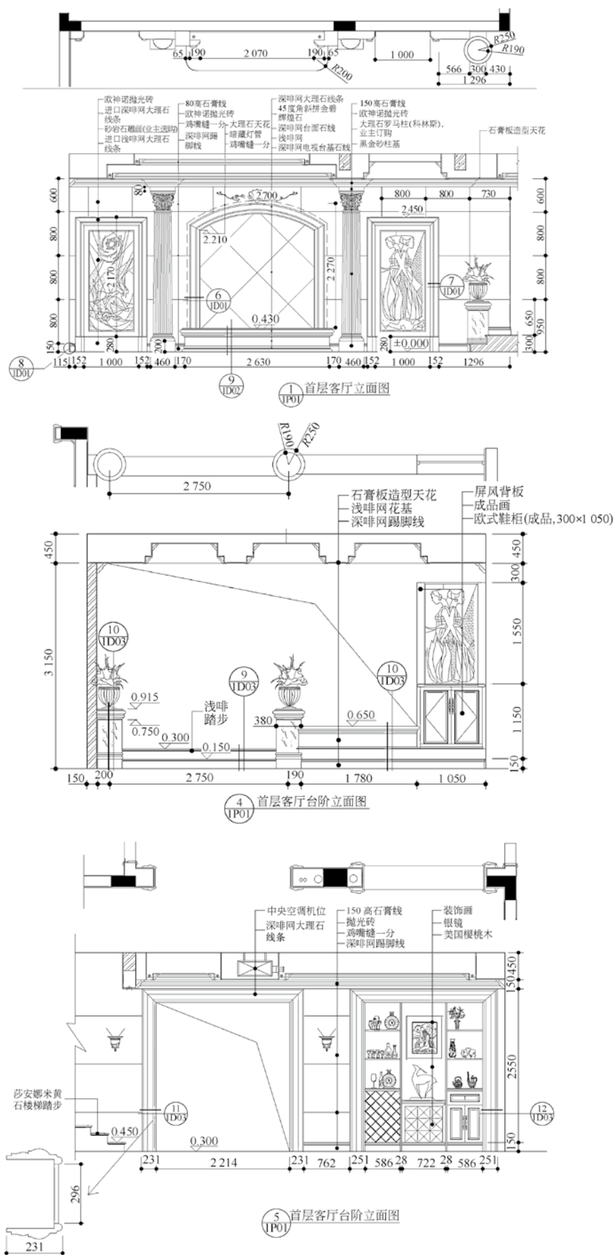
图 1-11 别墅设计立面图 (1) (文健、石树勇 设计)
