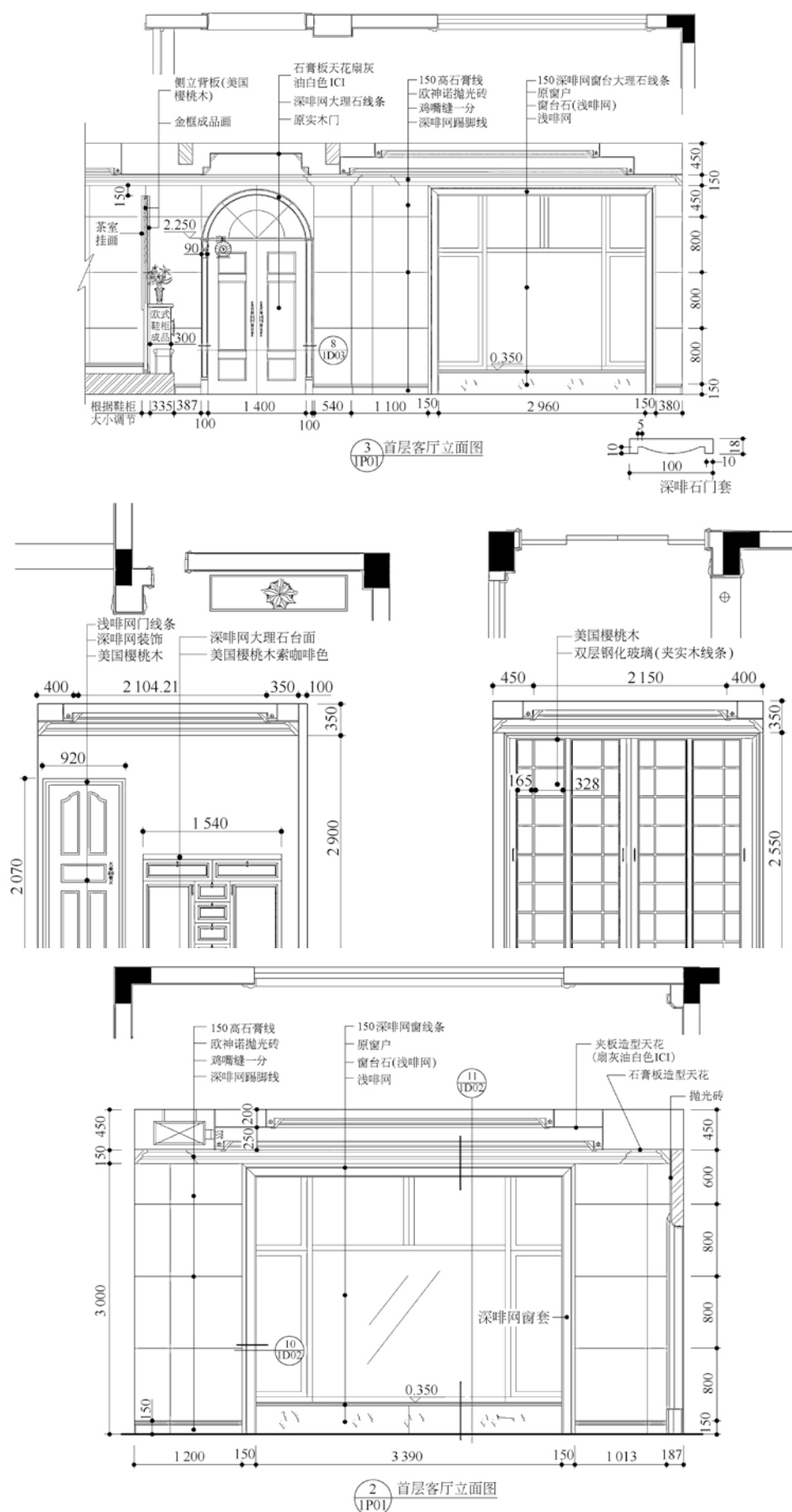
图 1-12 别墅设计立面图 (2) (文健、石树勇 设计)
