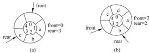
图 3-8 队列长度判断
