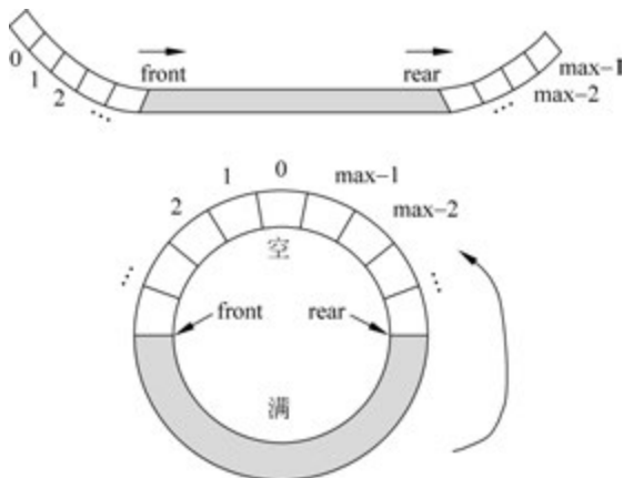
图 3-6 循环队列的逻辑结构
