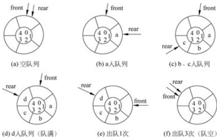
图 3-7 循环队列的入队和出队操作
