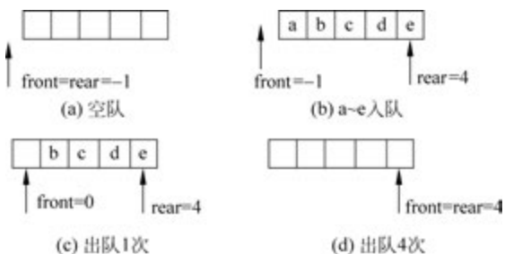
图 3-5 顺序队列的操作
